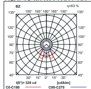
AGAT T5 4x14W PPAR-P RR
