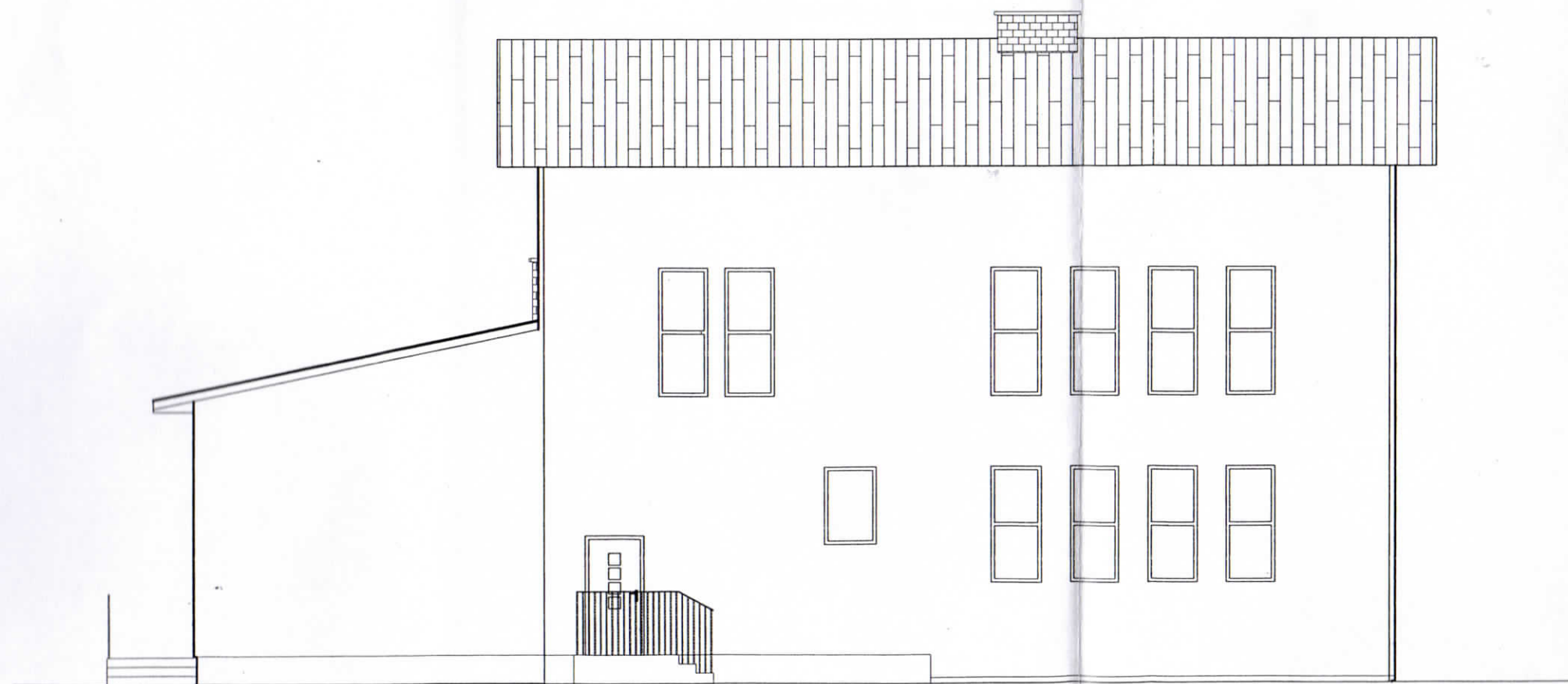
ELEWACJA ZACHODNIA
