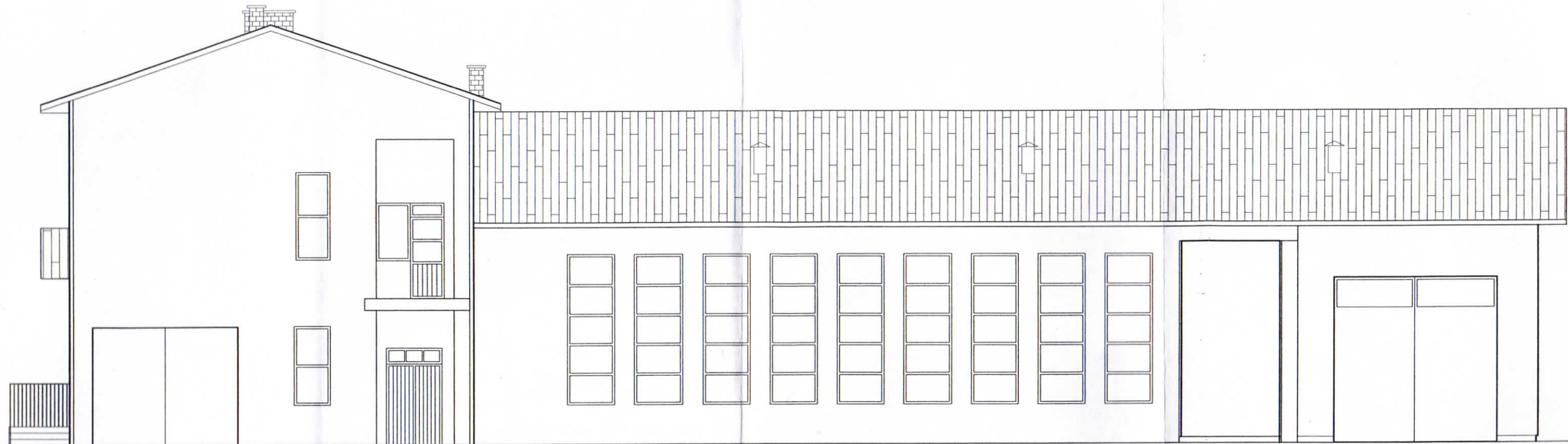
ELEWACJA POŁUDNIOWA
