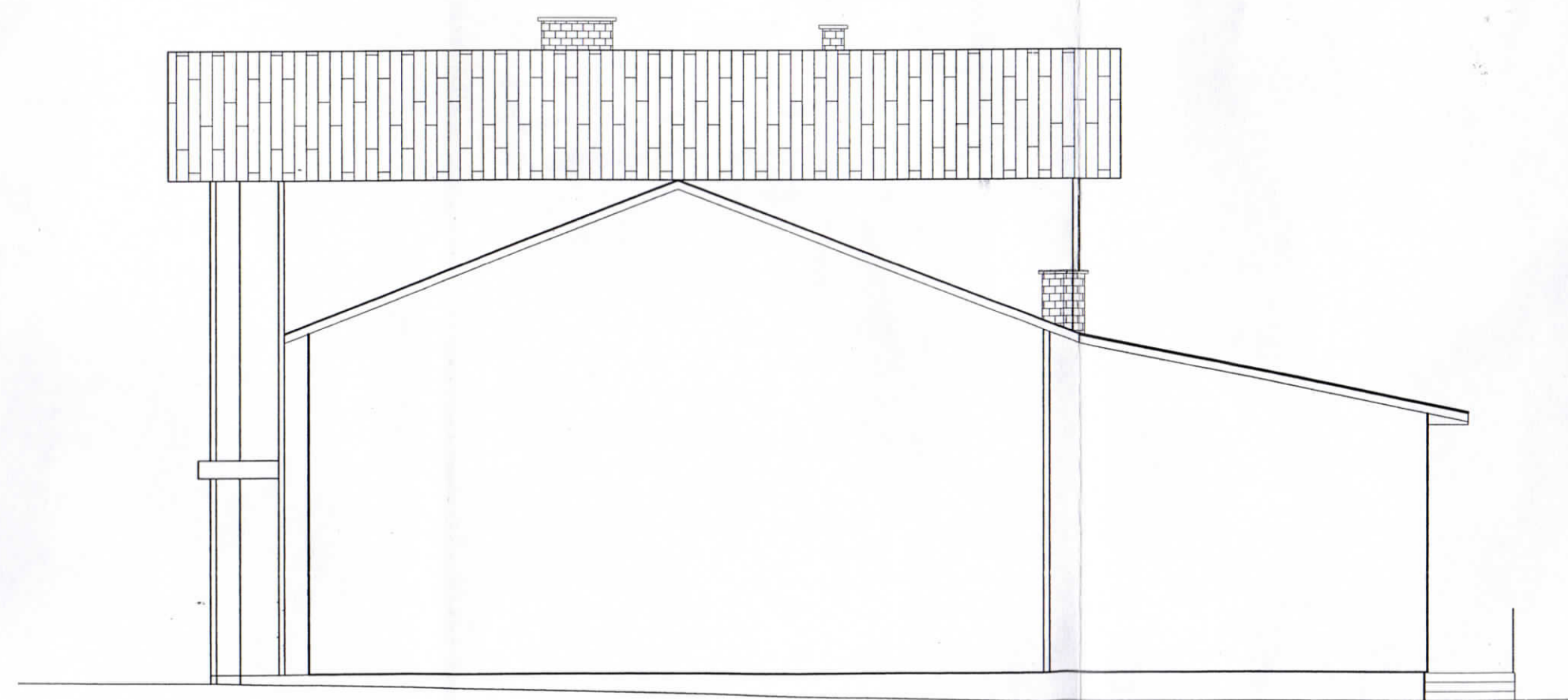
ELEWACJA WSCHODNIA
